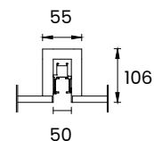
Trave da incasso registrabile
